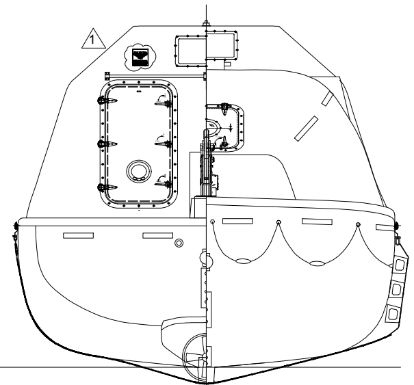
REAR/FRONT VIEW
